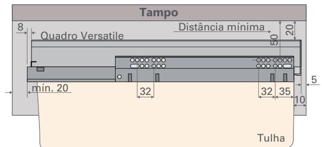
VISTA LATERAL
