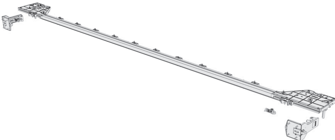
Trilho inferior
